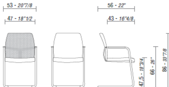
EASY-B, cantilever con schienale in rete o imbottito.
